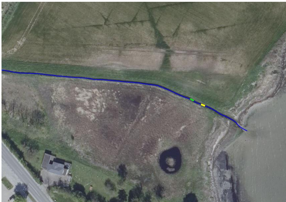
Figur 2: Luftfoto, der viser nuværende overkørsel som nedlægges og fjernes (markeret med grøn) og omtrentlig placering af ny overkørsel (markeret med gul). Lundby Bæks forløb er markeret med blå.
